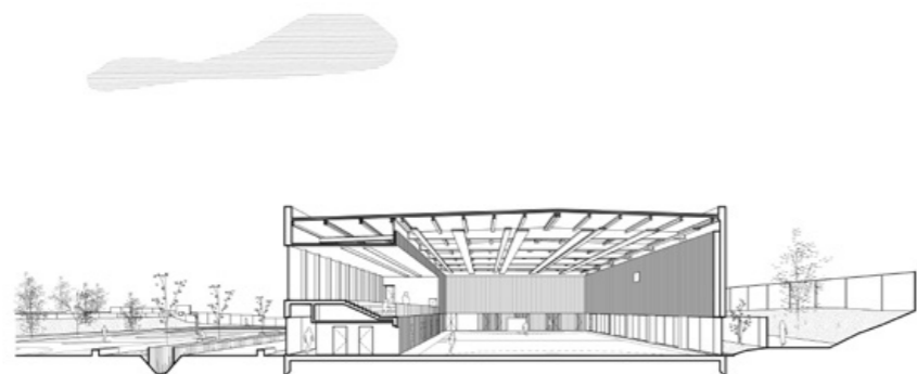
Coupe perspective transversale
