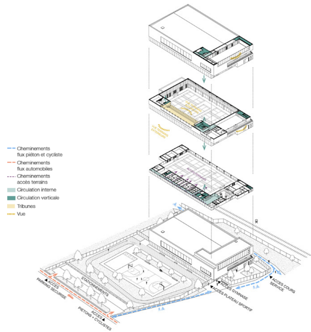
Axonométrie fonctionnelle
